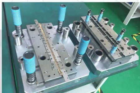
Khuôn dập Stamping mold
