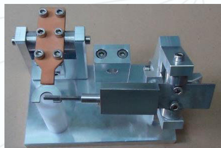
Đồ gá, dưỡng kiểm Jigs calibs
